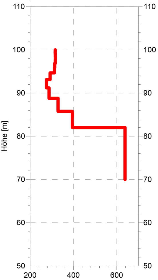
S - Wellengeschwindigkeit Oberflächenwellenseismik
