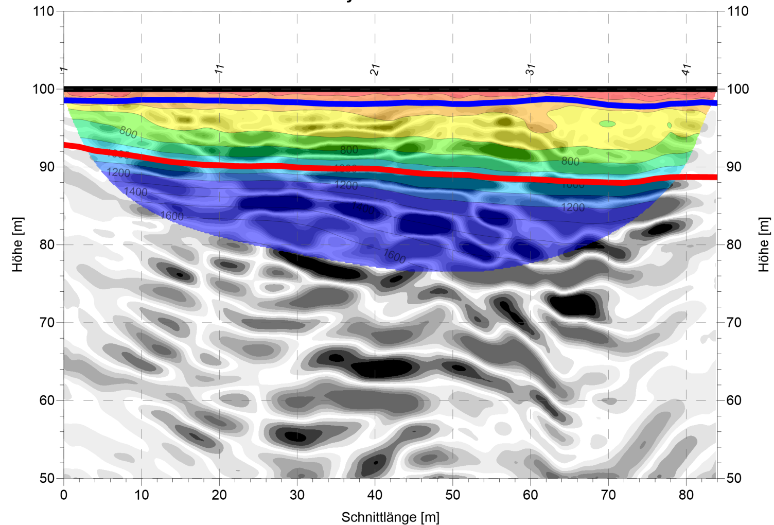
Hybridseismik
