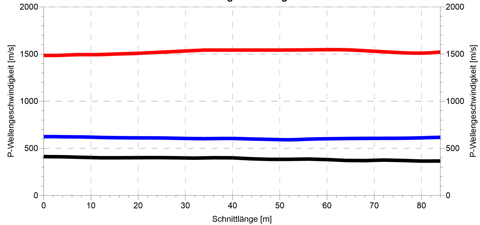
P - Wellengeschwindigkeit
